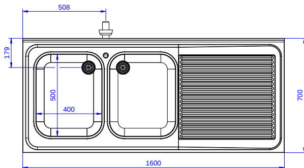
Boven aanzicht
