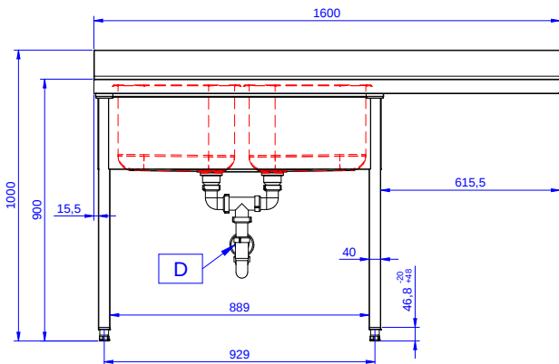
Zij aanzicht
